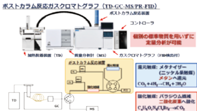
定量的ノンターゲット分析 (qNTA) に用いる ポストカラム反応ガスクロマトグラフ (TD-GC-MS/PR-FID)
