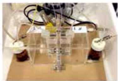
細胞から抽出した膜を用いて電解質、栄養素、薬物等の輸送を評価する ユッシングチャンバーシステム
