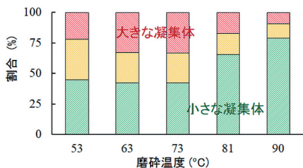
様々な温度で磨砕して調製した豆乳中のタンパク質凝集体の分画
