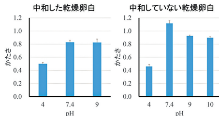
乾燥卵白から調製した泡のかたさに対するpHの影響
